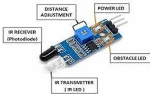
Fig. IR Sensor
